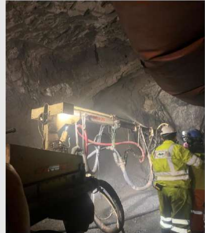
LANZADO DE SHOTCRETE EN VIA HUMEDA
